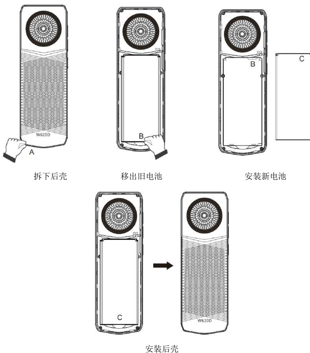
图 2 - 更换电池
