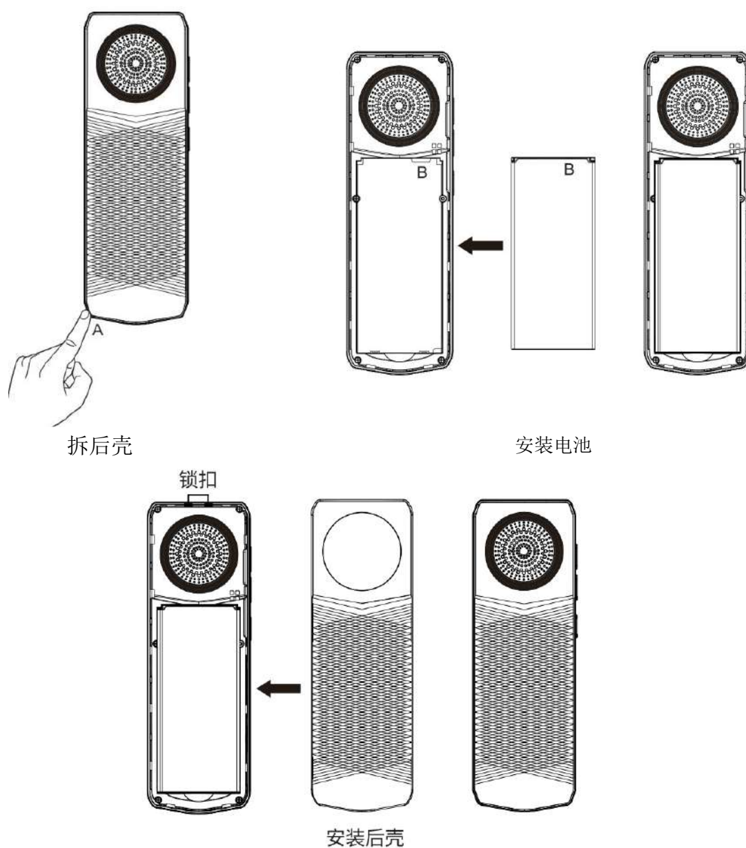
图 1 - 安装电池
